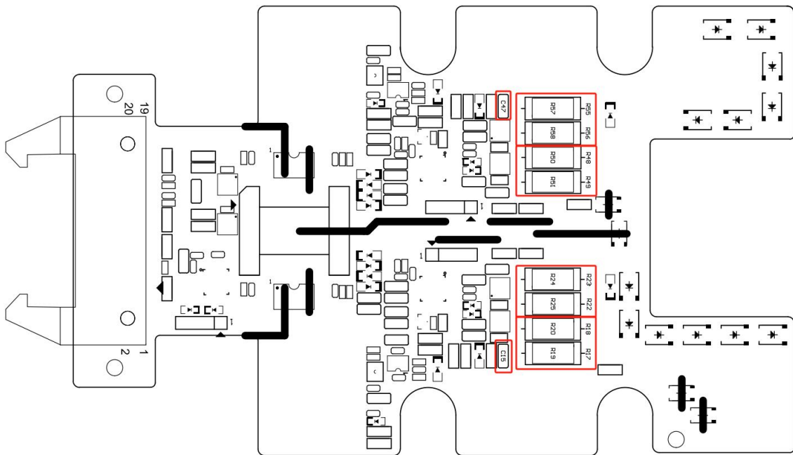
门极电阻电容位置指示图
