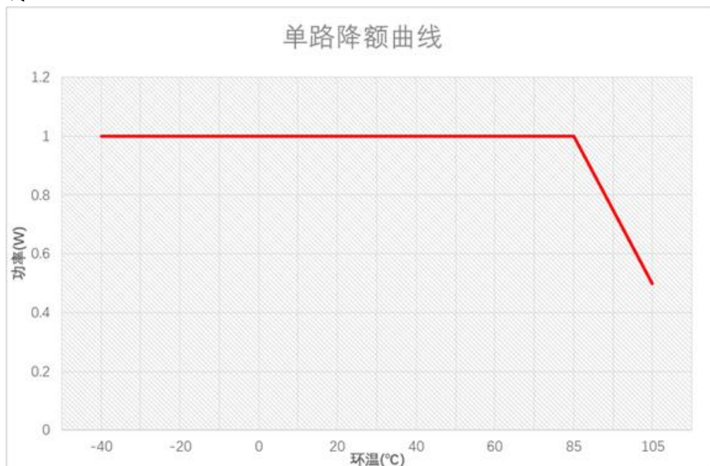
图 4 降额曲线图
