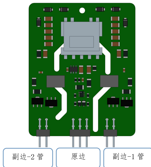
图 5 2FSC0110T12B1 驱动板原副边示意图
