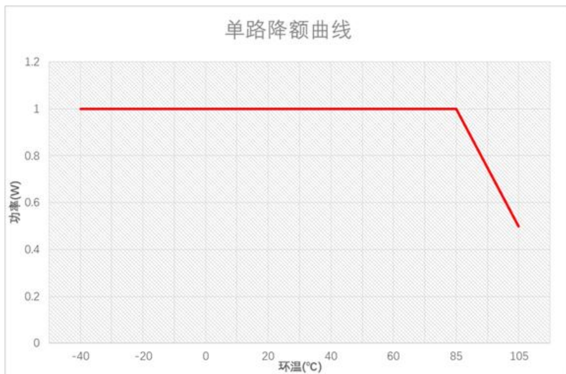
图 4 降额曲线图
