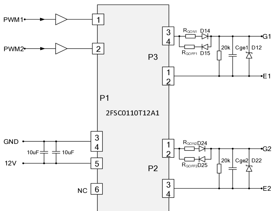
图 6 2FSC0110T12A1 典型应用图
