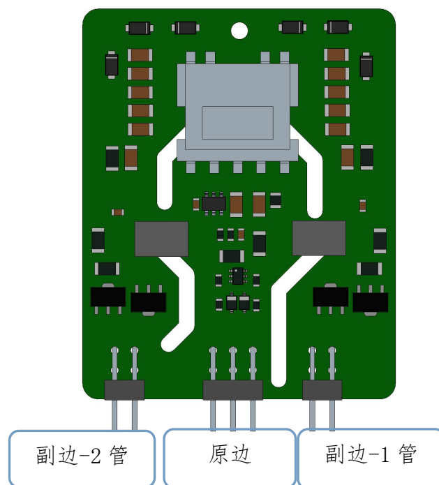
图5 2FSC0110T12A1 驱动板原副边示意图
